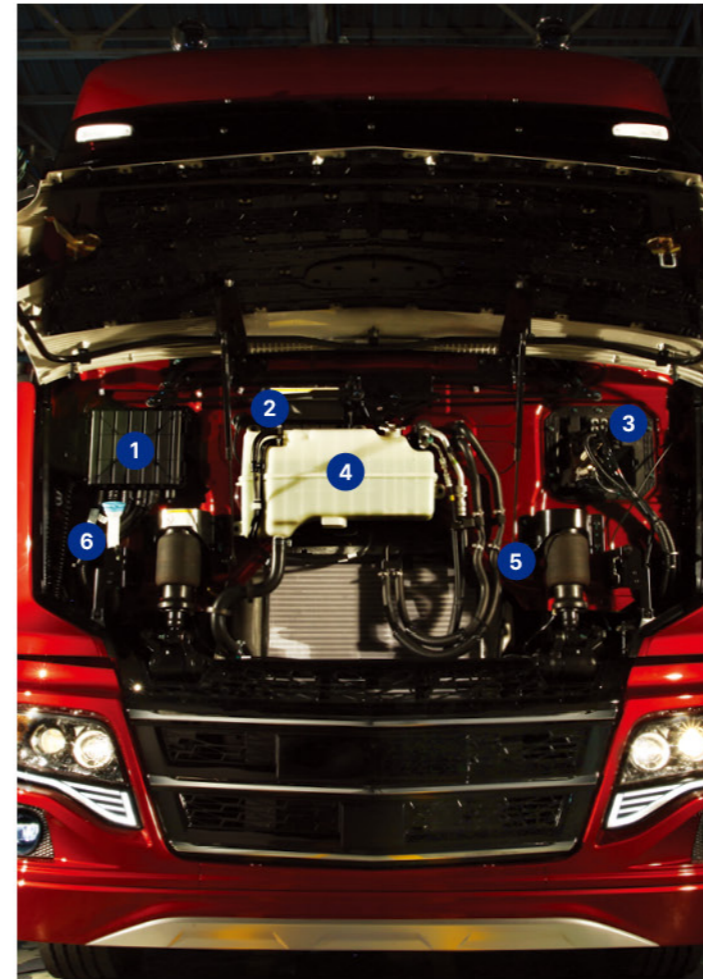
1 멀티 커넥터 3 브레이크 페달 모듈 5 전방 캡 서스펜션 2 에어컨 필터 4 냉각수 탱크 (서지탱크) 6 워셔액 주입구
